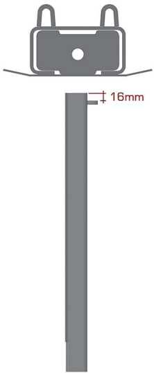
S-710 Fueiro Lateral Inferior
