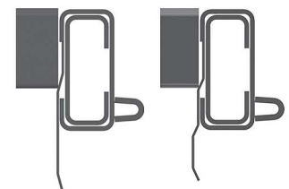
N-502 Batente Antigo
