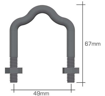
G-600 Presilha - mod.2011
