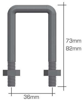
R-248-A Presilha da Tapa (82mm)
