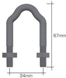
G-601 Presilha da Tapa - mod.2011
